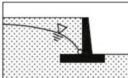
Joonis 20. Geosüntetide kasutamine drenaažisüsteemides
