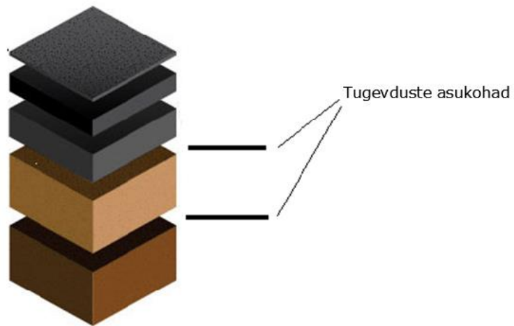
Joonis 13. Geosünteetide asukohad kandevõime parandamiseks
