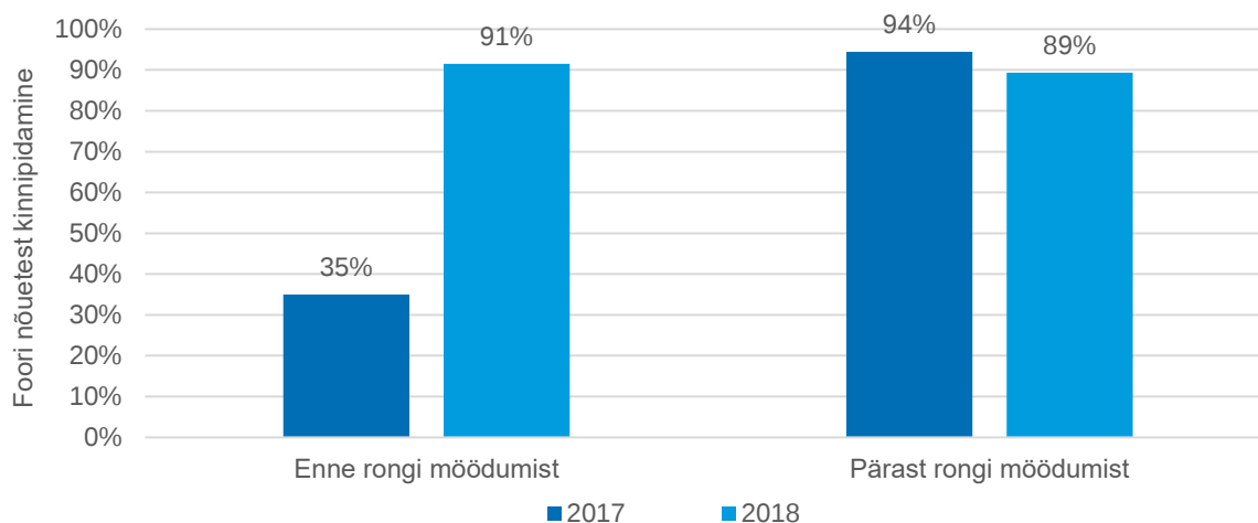
Joonis 26. Ainult fooriga varustatud raudteeülesõidukoha nõuete järgimise muutus 2017-2018.
