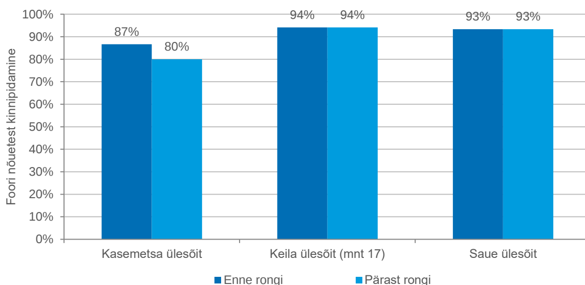
Joonis 23. Foori nõuetest kinnipidamine fooritsükli alguses ja lõpus.
