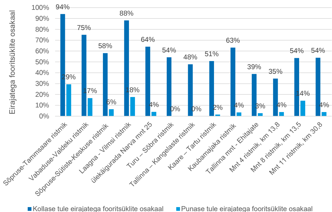
Joonis 2. Eirajatega fooritsüklite osakaal vaatluskohtade lõikes
