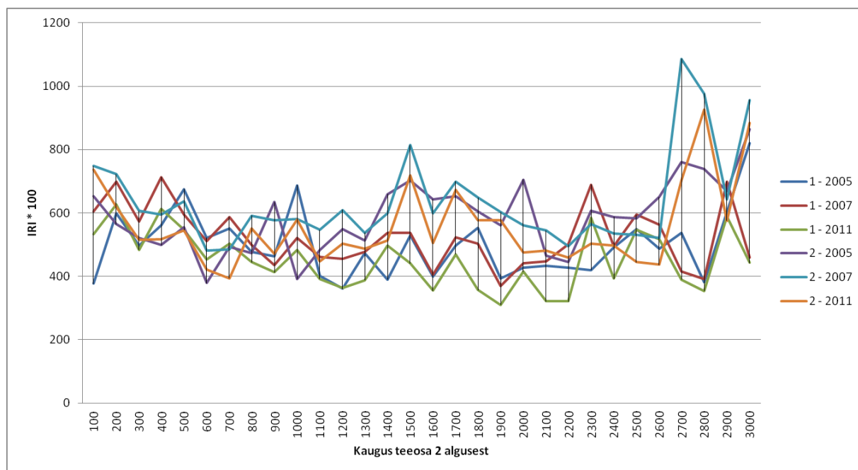
Joonis 5. Tasasus objekti piirkonnas teosal 2
