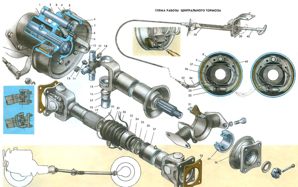
Joonis 1 - GAZ 21 seisupiduri tsentraalam. Allikas: http://gaz21.tut.nov.ru/system/files/images/album/020.jpg
